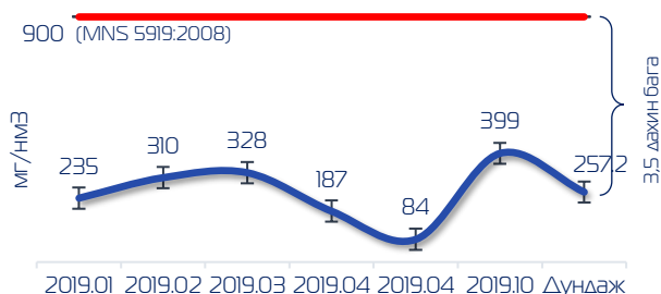
Цахилгаан станцын утааны хийн найрлага дахь NO x
